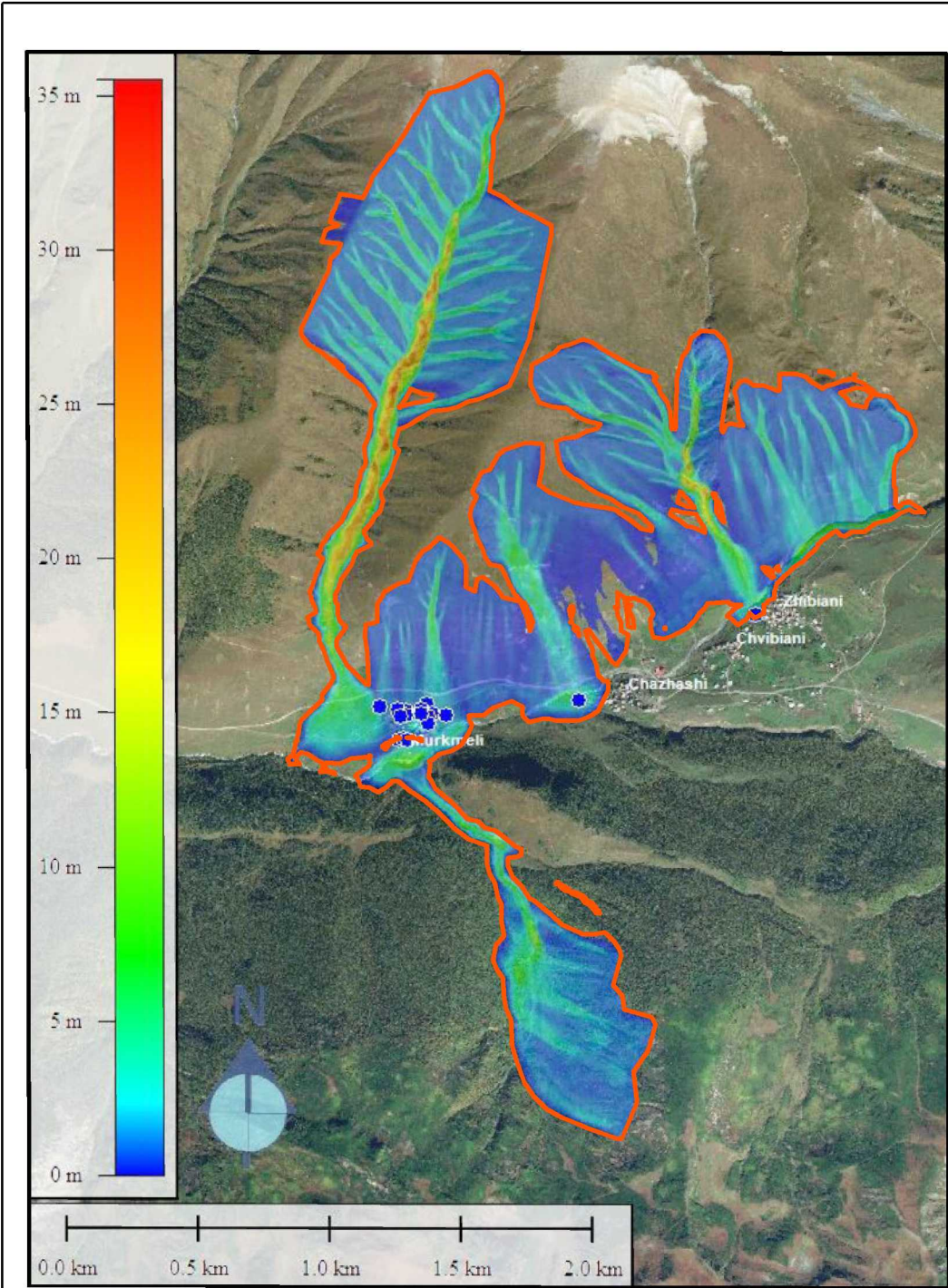
100 წლიანი განმეორებადობის ზვავის Ramms მოდელირება - მაქსიმალური სიმაღლე Ramms modeling of potential 100 years return period avalanche – maximum height
