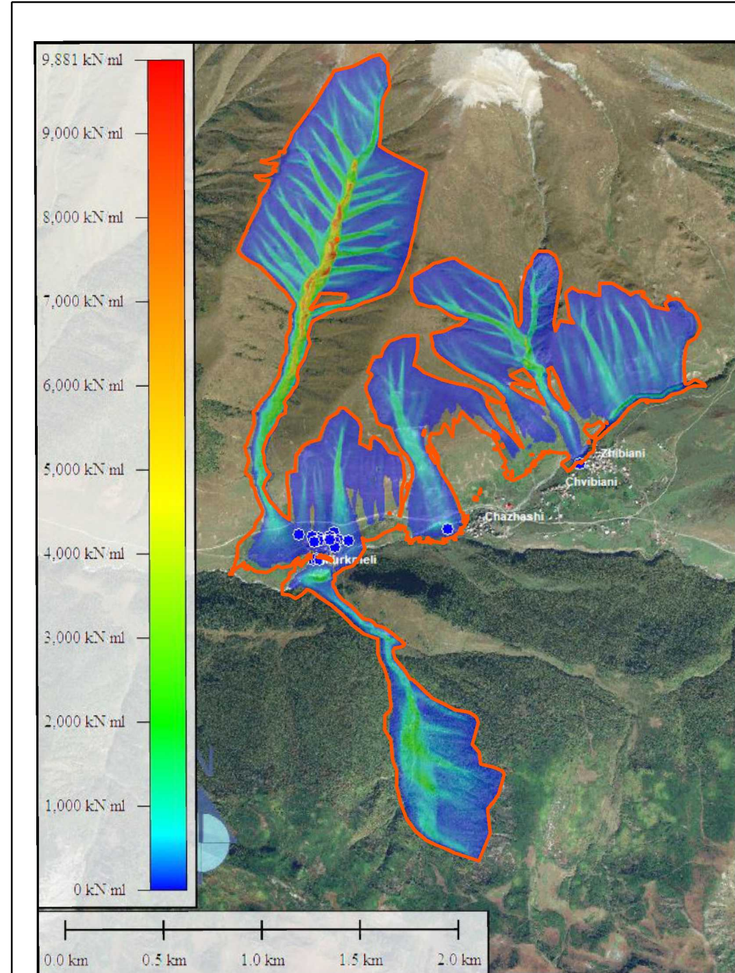
100 წლიანი განმეორებადობის ზვავის Ramms მოდელირება - ზვავის ინტენსივობა Ramms modeling of potential 100 years return period avalanche – avalanche intensity
