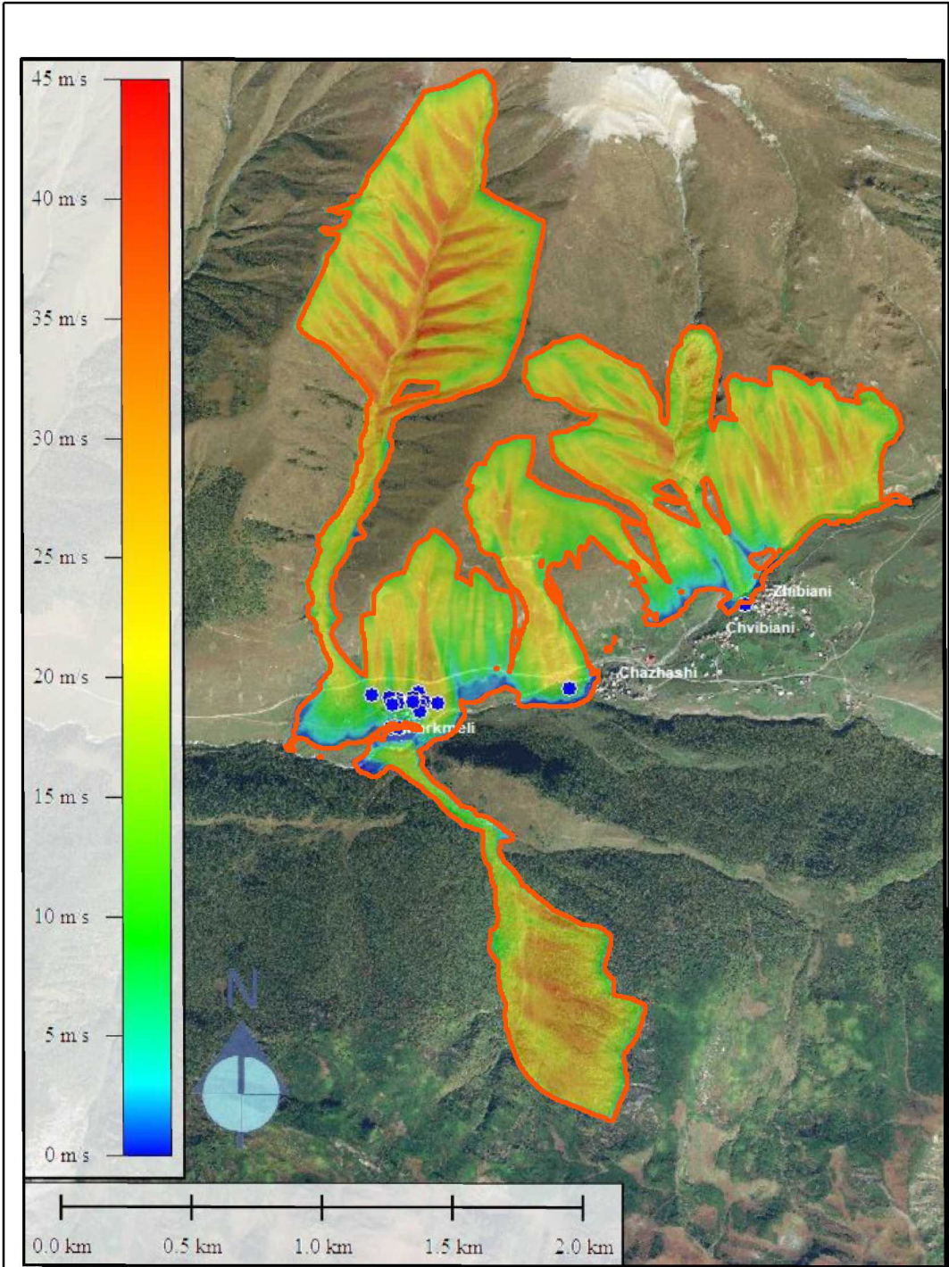
100 წლიანი განმეორებადობის ზვავის Ramms მოდელირება - მაქსიმალური სიჩქარე Ramms modeling of potential 100 years return period avalanche – Maximum speed
