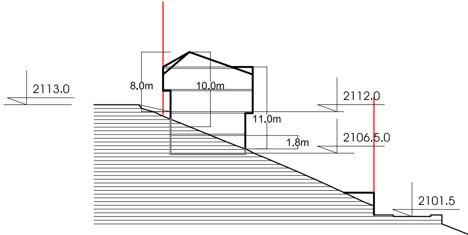
პროექტი 2-2
