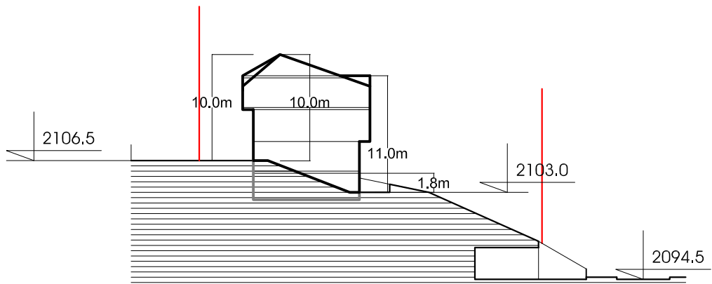
პროექტი 1-1
