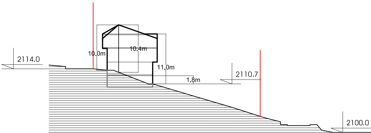
პროექტი 3-3
